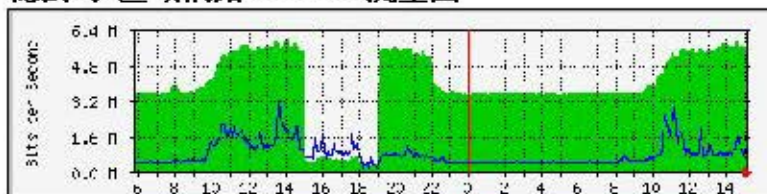
語音網管器 4M/1M adsl 流量圖
